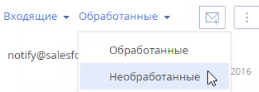
Рис. 192 — Выбор фильтра
