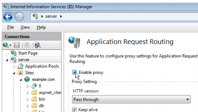
Рис. 532 — Включение прокси
