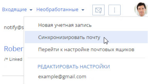
Рис. 191 — Синхронизация почты
