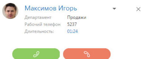
Рис. 216 — Идентификация абонента
