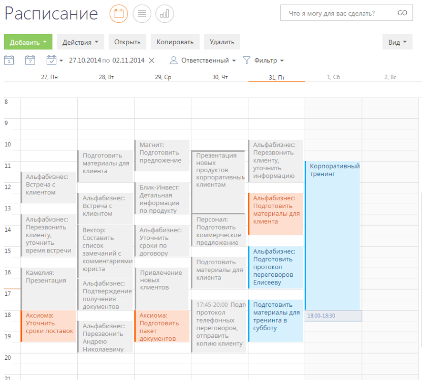
Рис. 269 — Представление [Расписание]
